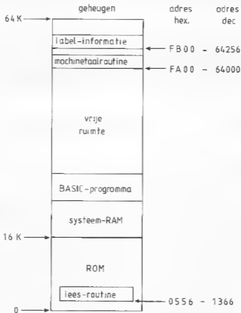
Afb. 6-2 Geheugenindeling na laden labelinformatie
